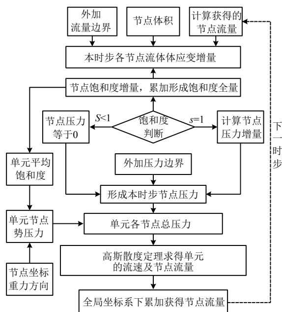
图1 渗流求解流程
