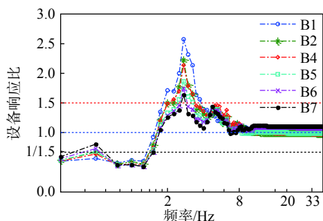
图 13 设备响应比
