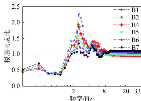
图 12 楼层响应比
