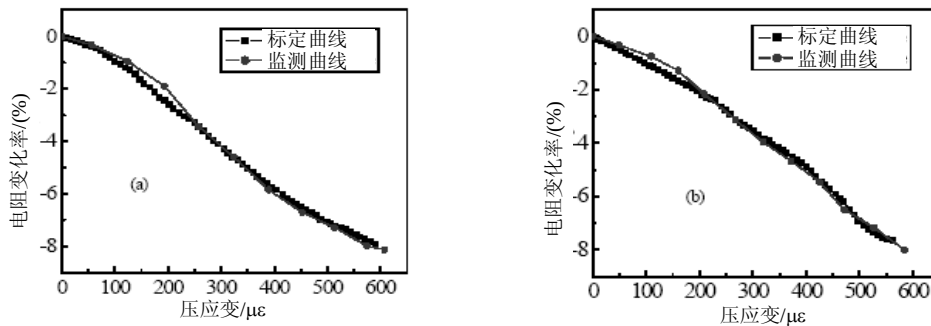
图 24 碳纤维水泥石压敏传感器压应变监测曲线与标定曲线的比较
