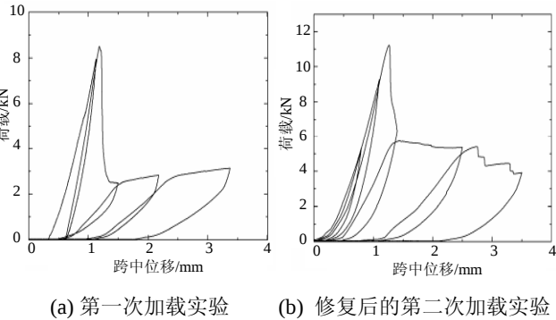
图 31 混凝土梁的荷载与跨中挠度曲线
