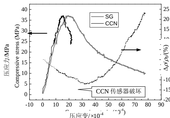
图 10 C40 混凝土柱在加载过程中由 CCN 传感器测得的应力-应变全曲线
