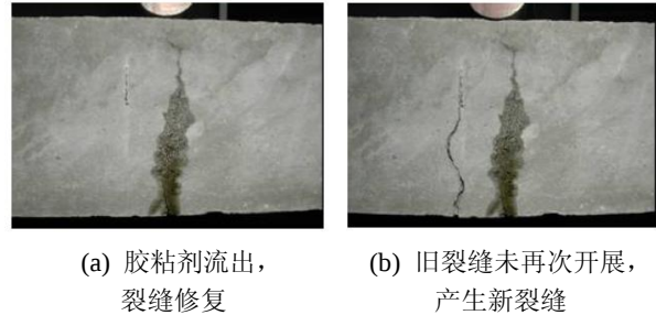
图 30 裂缝的开展及修复图
