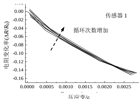
图 8 CCN 传感器在幅值 10kN 循环荷载下的应变感知特性曲线
