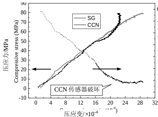
图 11 C80 混凝土柱在加载过程中由 CCN 传感器测得的应力-应变全曲线
