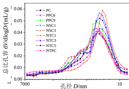
图5 混凝土的孔径分布微分曲线
