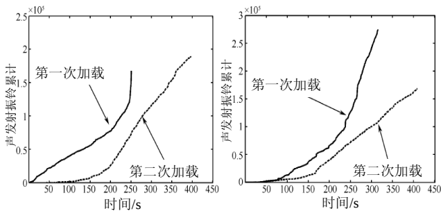
图 32 未修复试件的声发射图
