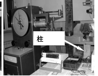
图 23 柱加载图
