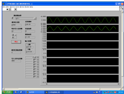
图 26 三点弯曲梁数据采集界面
