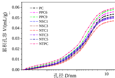
图4 混凝土的孔径分布积分曲线
