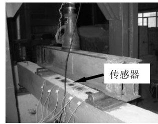
图 22 梁加载图
