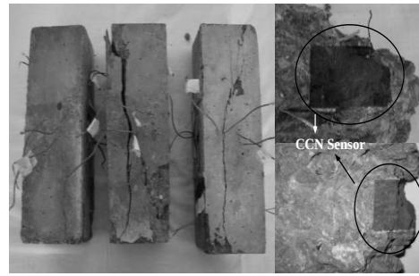
图 13 破坏后的 C80 混凝土柱及其内的 CCN 传感器
