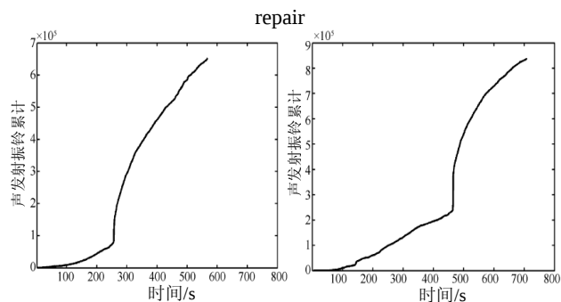
图 33 修复试件修复前后的声发射图
